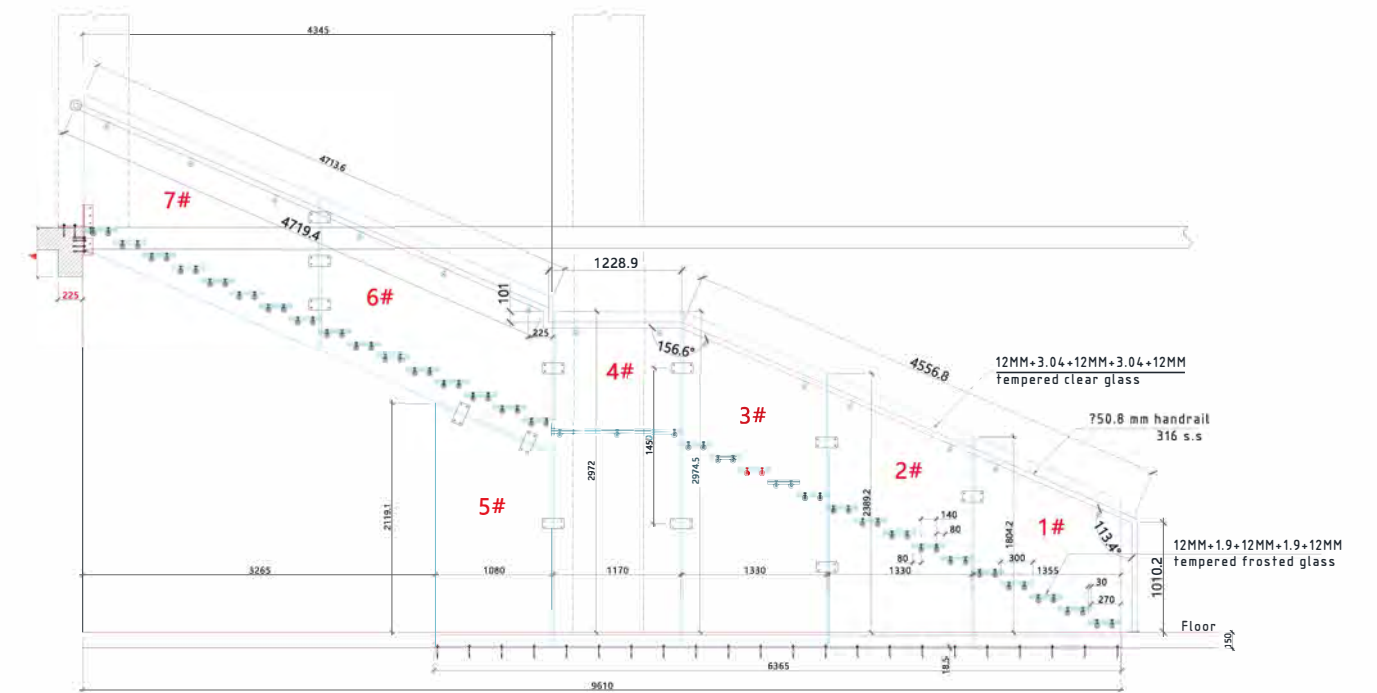
B ELEVATION
