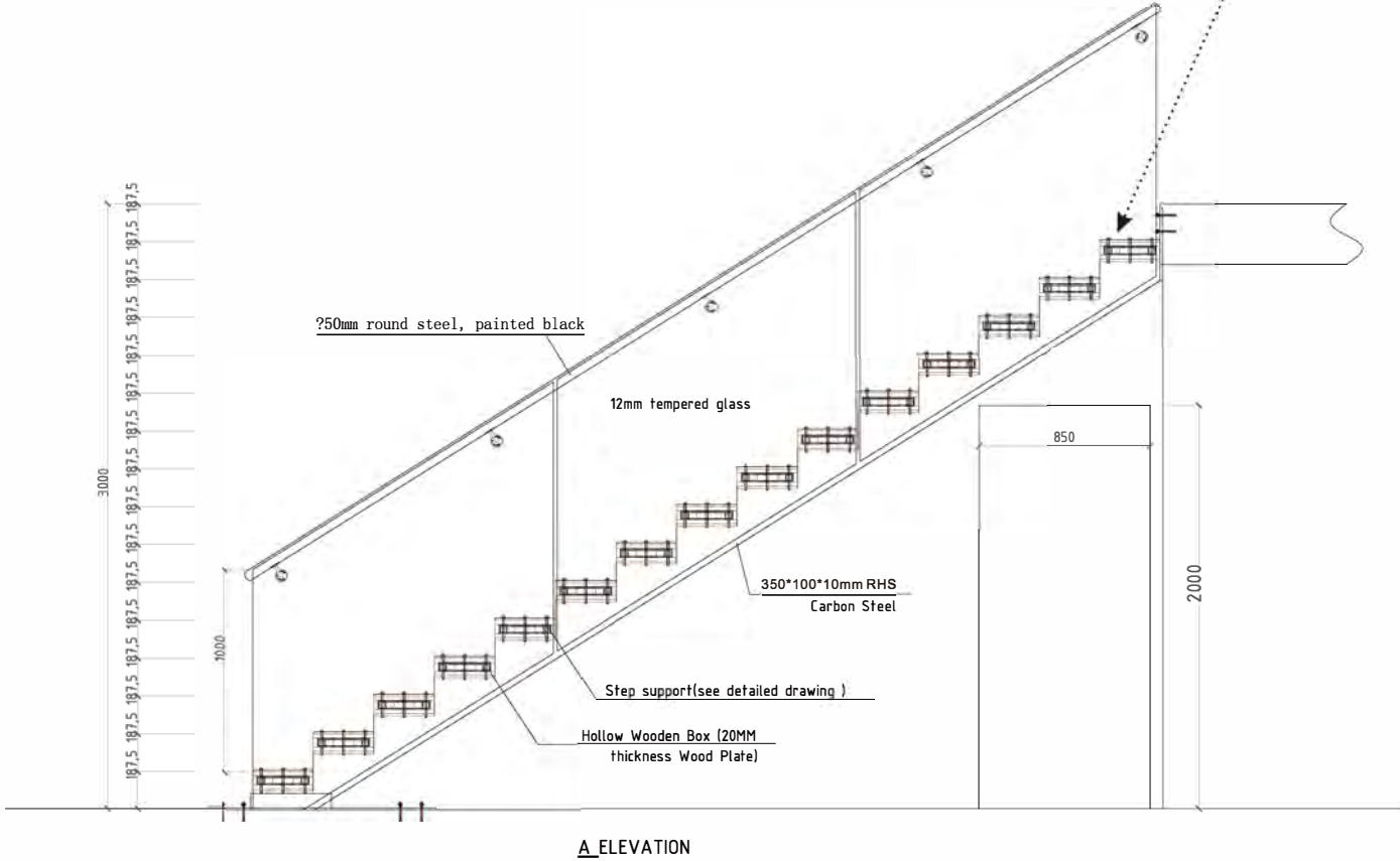
A ELEVATION
