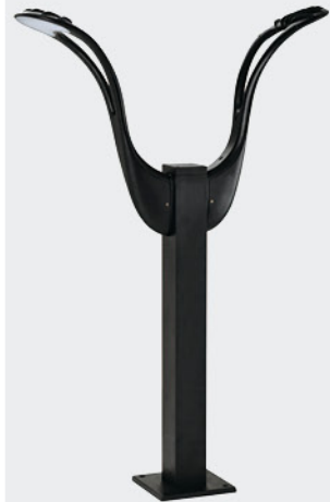
GMD-F823-2-90CM SMD:2 × 10W Size:150 × 640 × 900
